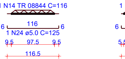
VT407a (3 unidades) (L407) ESC 1:50
