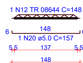
VT510a (11 unidades) (L510) ESC 1:50
