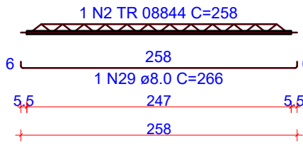
VT405a (1 unidades) (L405) ESC 1:50
