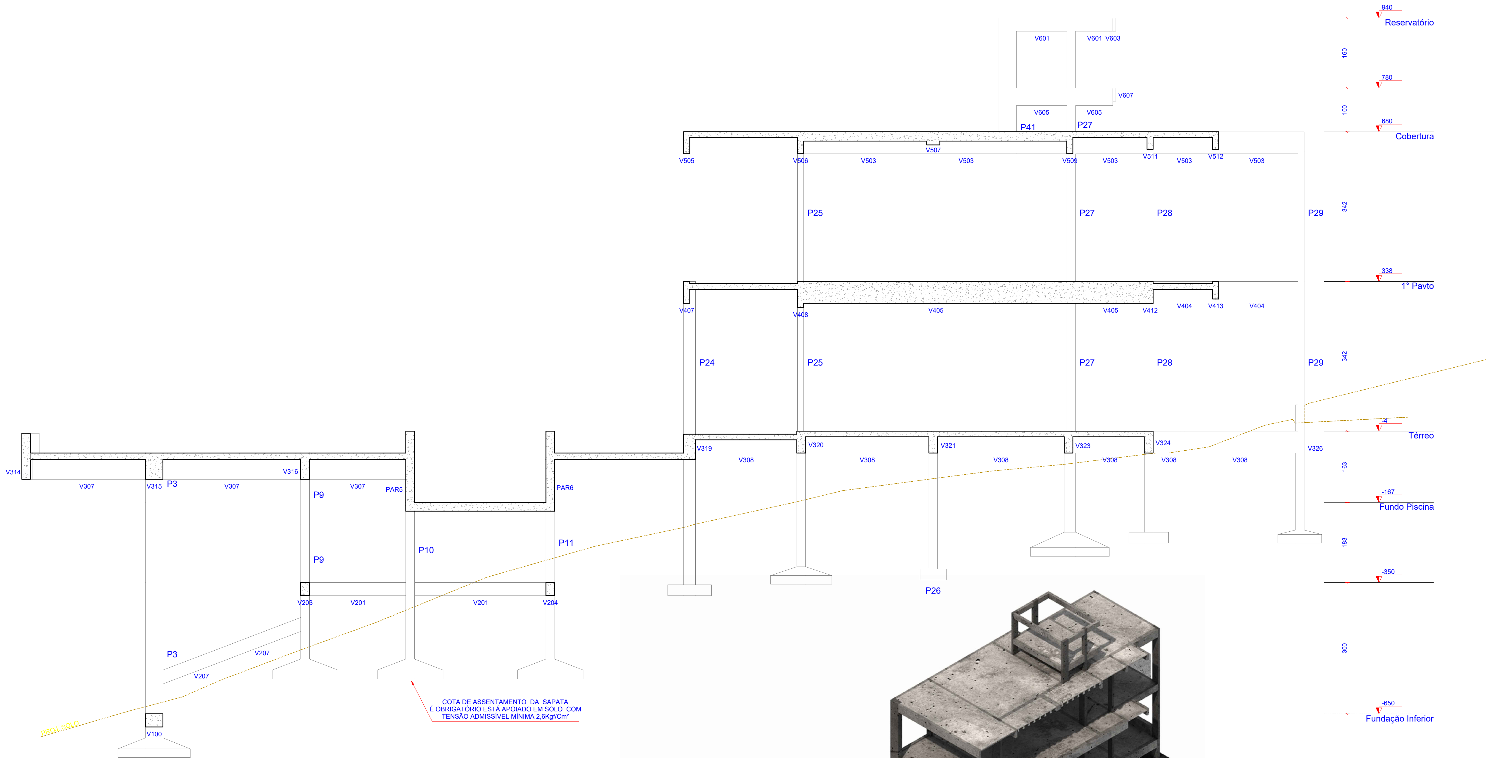
1 CORTE E-E ESCALA 1:50
