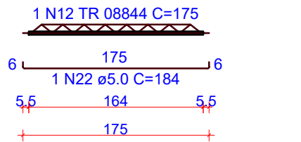
VT406b (4 unidades) (L406) ESC 1:50
