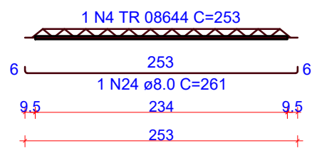
VT500d (1 unidades) (L500) ESC 1:50
