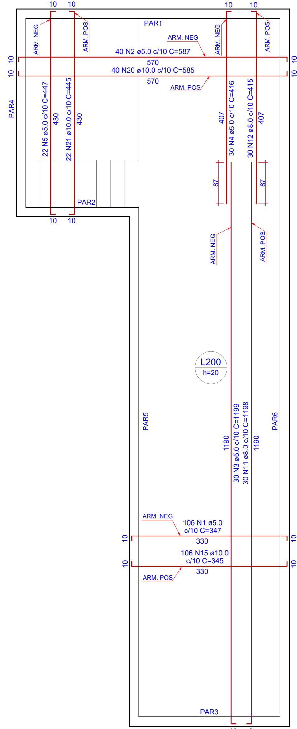
ARMADURA POSITIVA E NEGATIVA DA LAJE - FUNDO PISCINA
