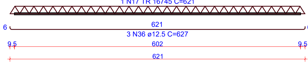
VT406c (1 unidades) (L406) ESC 1:50
