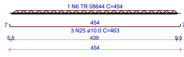
VT504a (5 unidades) (L504) ESC 1:50
