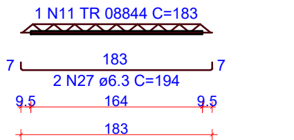
VT406a (3 unidades) (L406) ESC 1:50
