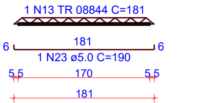
VT406c (1 unidades) (L406) ESC 1:50
