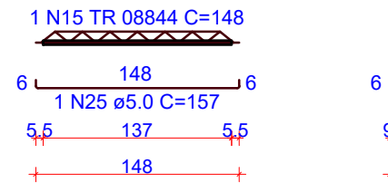
VT408a (4 unidades) (L408) ESC 1:50
