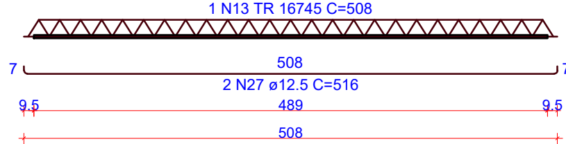
VT501a (10 unidades) (L501) ESC 1:50
