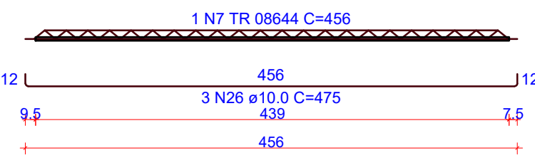
VT504b (3 unidades) (L504) ESC 1:50
