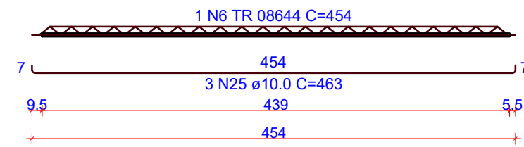
VT504c (2 unidades) (L504) ESC 1:50
