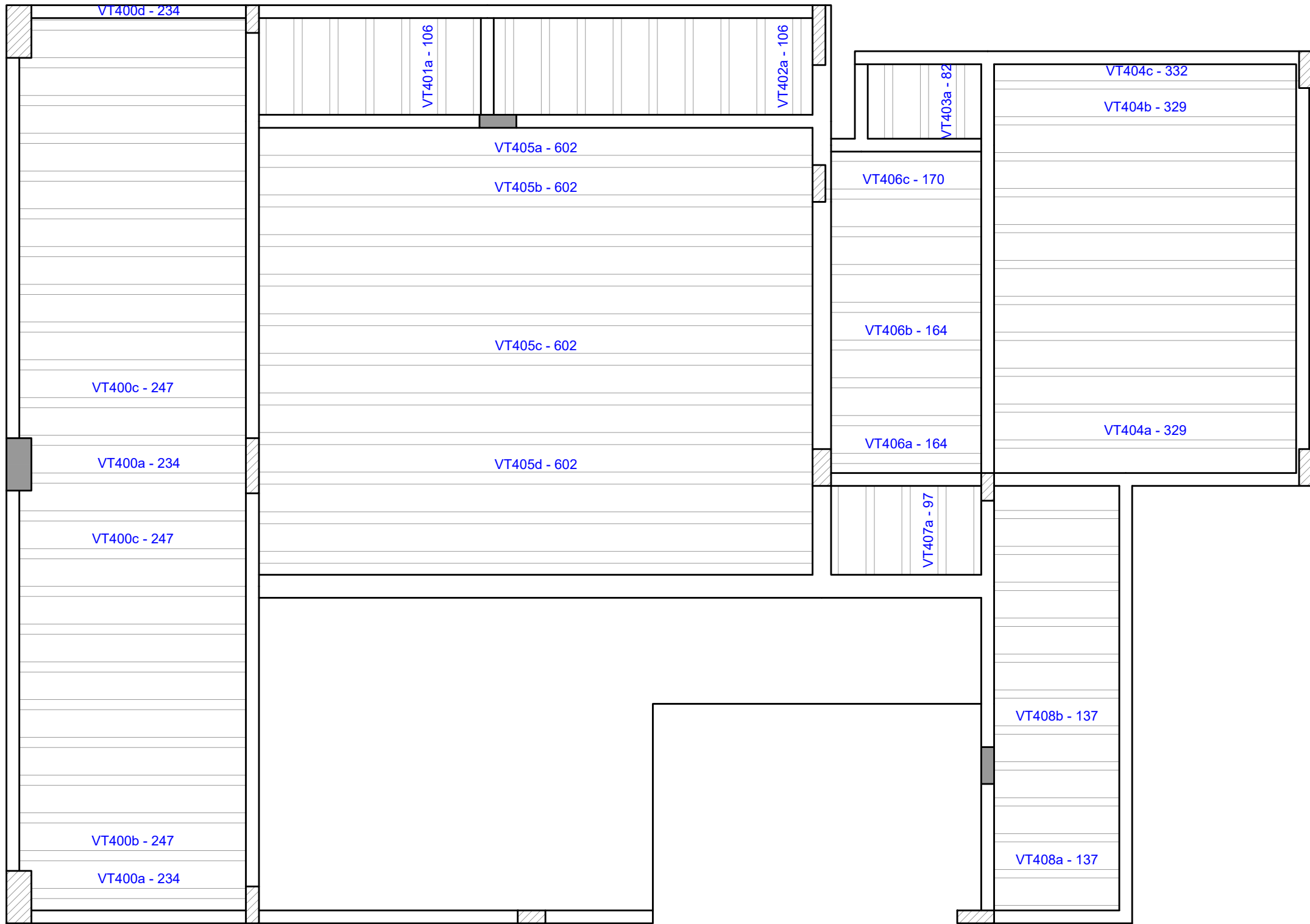
1 PLANTA DE VIGOTAS PRÉ-MOLDADAS - 1º PAVIMENTO ESCALA 1:50
