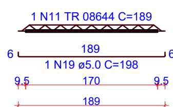
VT509a (13 unidades) (L509) ESC 1:50
