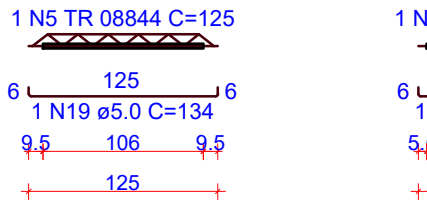
VT401a (5 unidades) (L401) ESC 1:50
