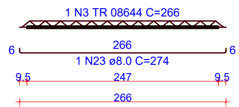
VT500c (10 unidades) (L500) ESC 1:50
