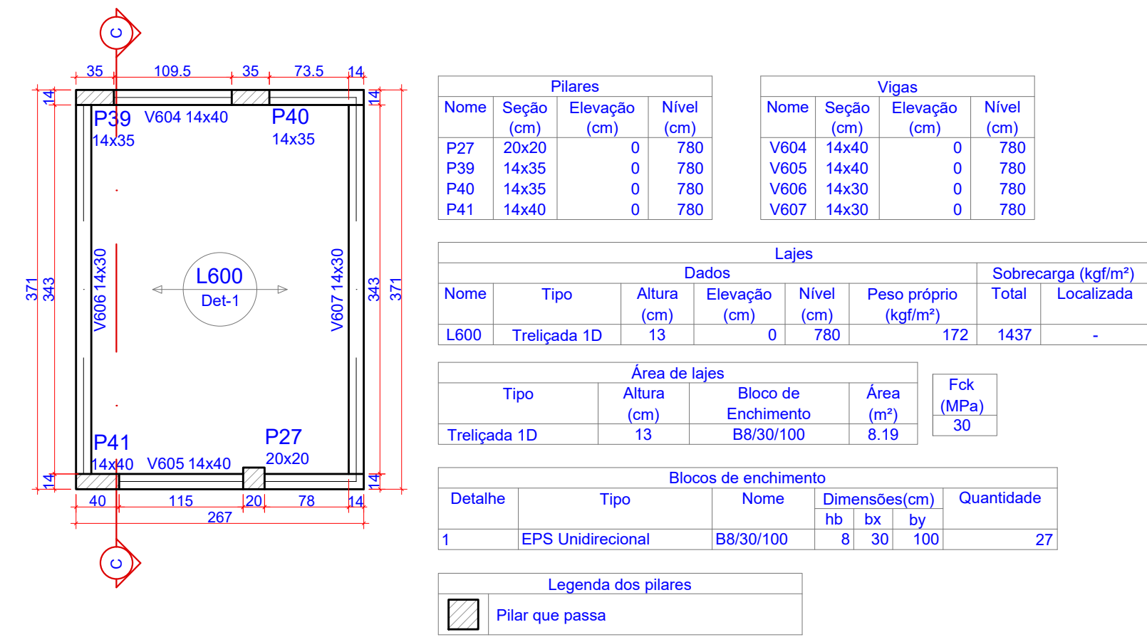
1 PLANTA DE FORMAS - INTERMEDIÁRIA RESERVATÓRIO (NÍVEL 780) ESCALA 1:50
