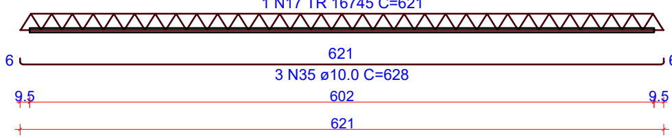
VT405c (3 unidades) (L405) ESC 1:50
