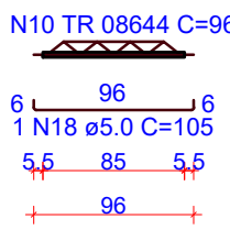
VT506b (7 unidades) (L506) ESC 1:50
