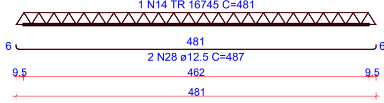
VT507a (14 unidades) (L507) ESC 1:50
