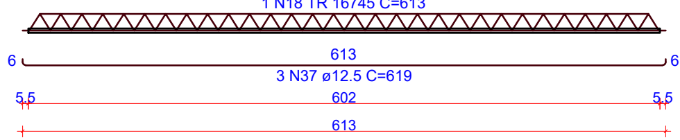
VT408a (4 unidades) (L408) ESC 1:50
