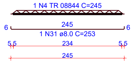
VT405b (4 unidades) (L405) ESC 1:50
