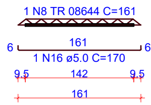
VT505a (8 unidades) (L505) ESC 1:50
