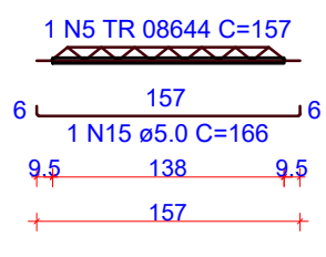
VT502a (3 unidades) (L502) ESC 1:50
