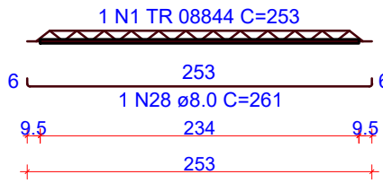
VT404c (1 unidades) (L404) ESC 1:50
