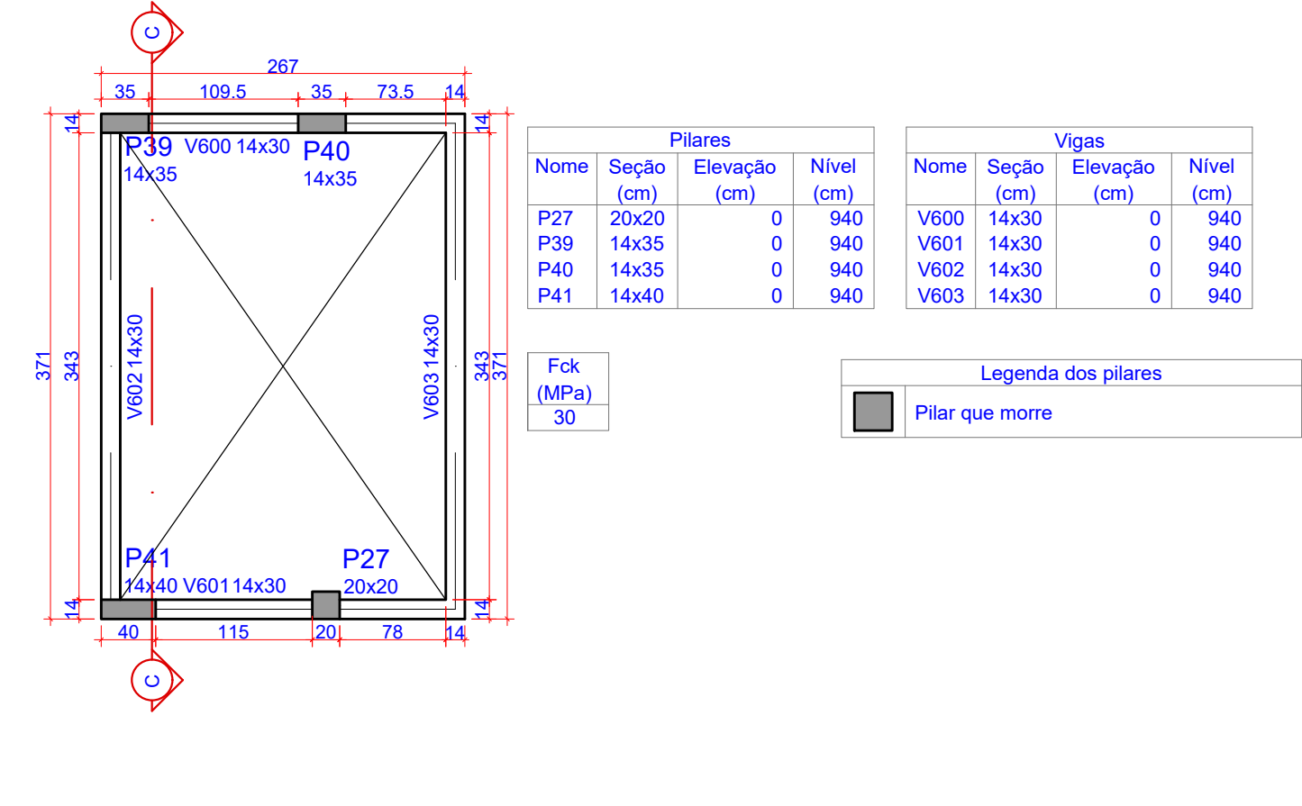
2 PLANTA DE FORMAS - TOPO RESERVATÓRIO (NÍVEL 940) ESCALA 1:50
