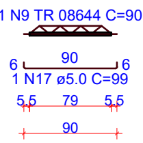
VT506a (1 unidades) (L506) ESC 1:50
