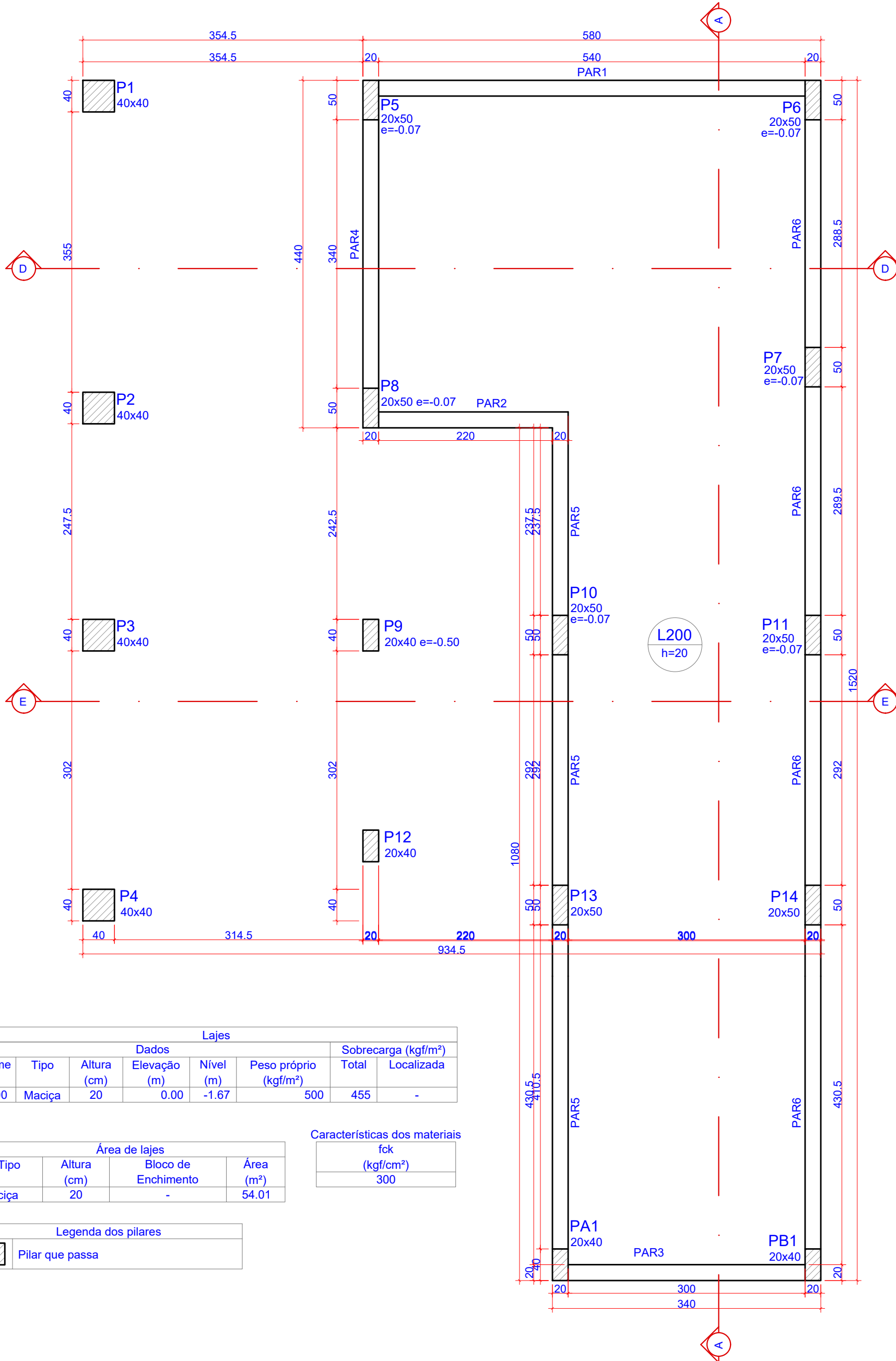
3 PLANTA DE FORMAS - FUNDO PISCINA (NÍVEL -167)
